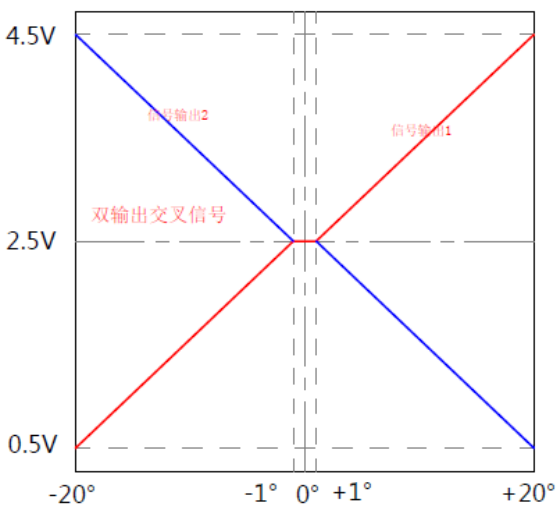
电压信号: 输出曲线三
