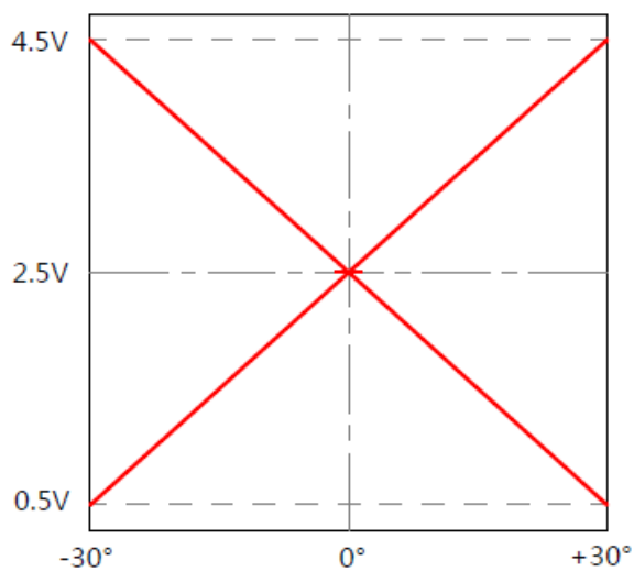
指拨轮输出曲线图2(双传感器)
