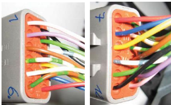
连接器背面图
