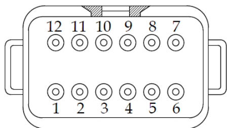
连接器背面图
