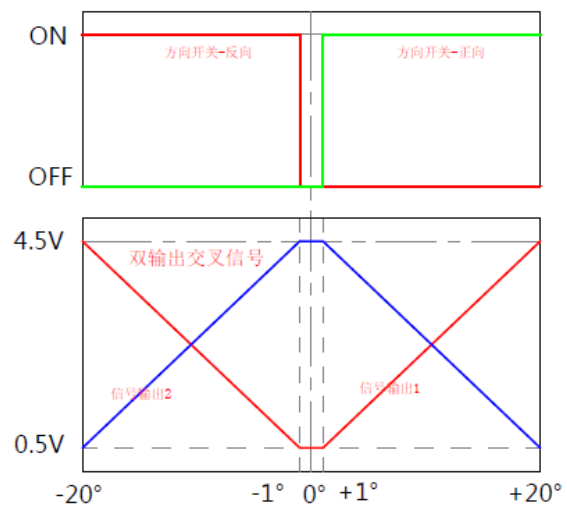
电压信号: 输出曲线四
