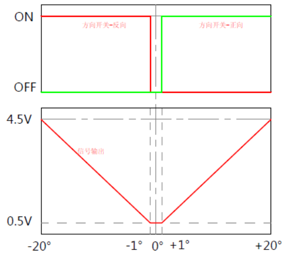
电压信号: 输出曲线二
