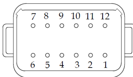
连接器正面图
