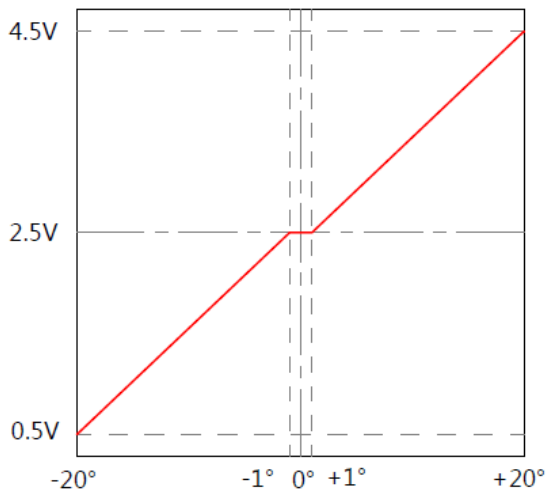
电压信号: 输出曲线一
